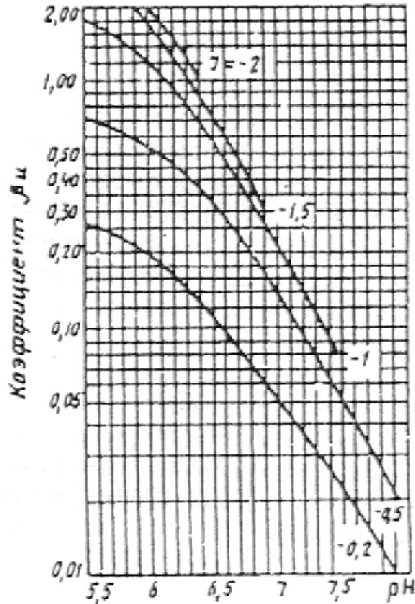
Рис. 4. Номограмма для определения коэффициента
