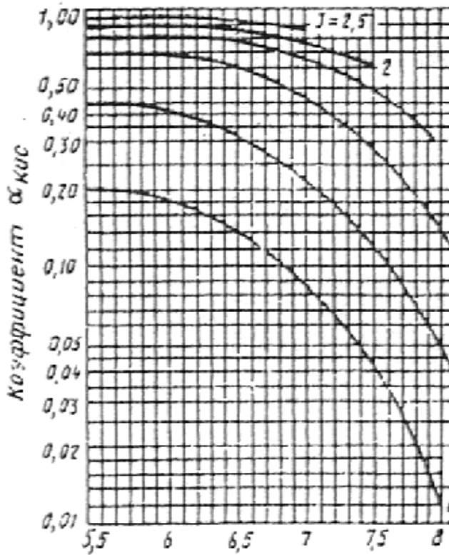
Рис. 3. Номограмма для определения коэффициента
