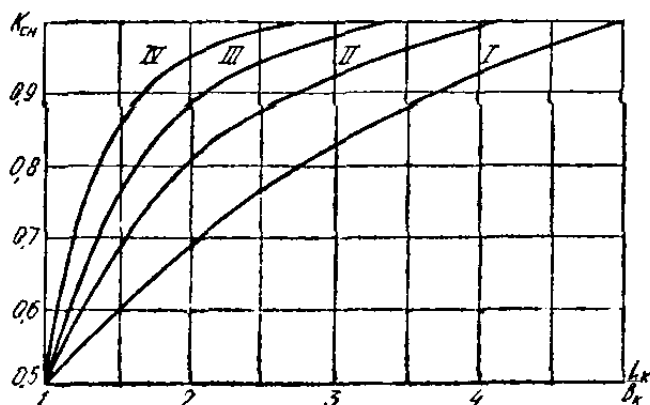
Рис. 6. Графики для определения коэффициента k_{сп} L_k - длина камеры; v_k - ширина камеры, I, II, III, IV - категории устойчивости пород
