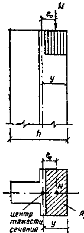
Рис. 5. Внецентренное сжатие
