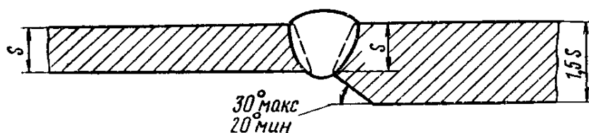
Рис. 1. Конструктивные размеры разделки кромок и сварных швов разнотолщинных труб (до 1,5 толщины стенки)
