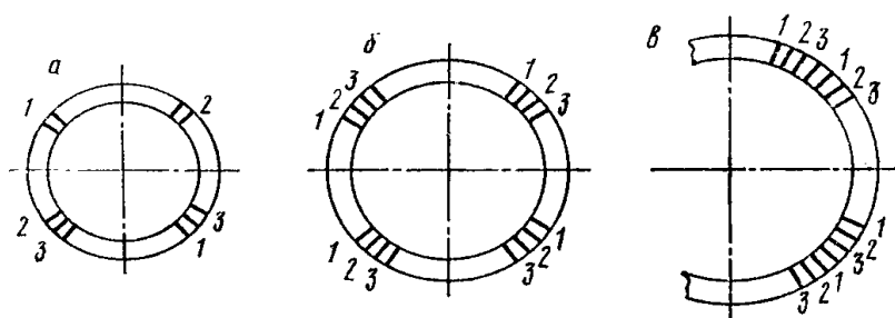
Рис. 3. Схема вырезки образцов для механических испытаний
