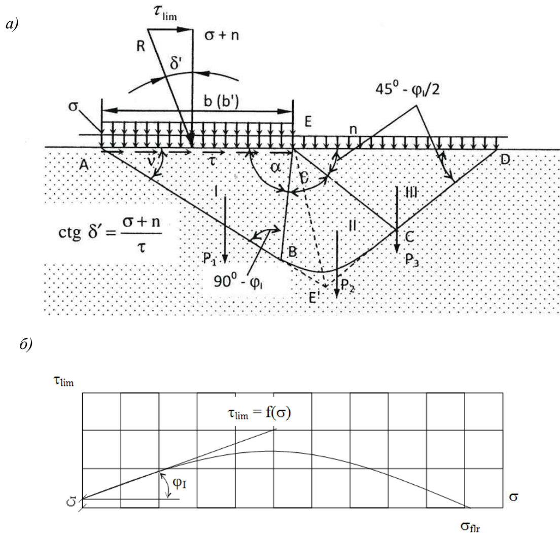
a – расчетная схема; б – график несущей способности основания; I, II, III – зоны призмы обрушения
