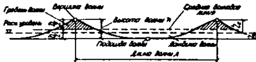
Профиль и элементы волны
