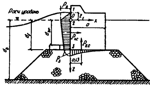
Рис. 8. Эпюры давления разбивающихся волн на вертикальную стену
