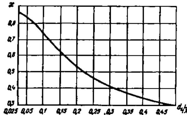
Рис. 32. График значений коэффициента \chi
