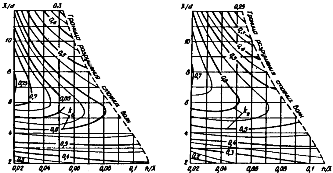
Рис. 5. Графики значений коэффициентов k_8 и k_9
