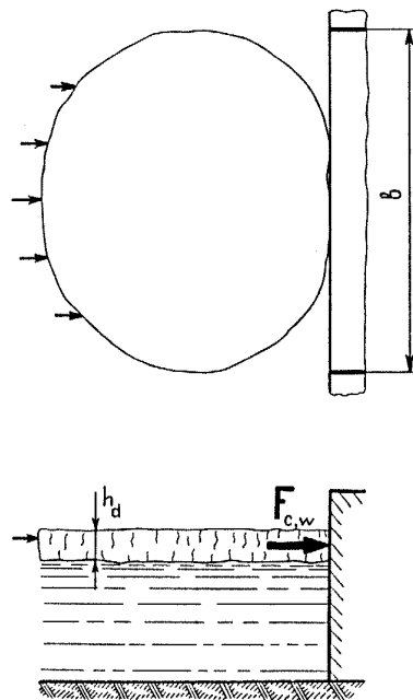
Рис. 36. Схема приложения нагрузки от движущегося ледяного поля на секцию сооружения
