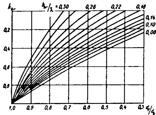
Рис. 2. Графики значения коэффициента k_{br}
