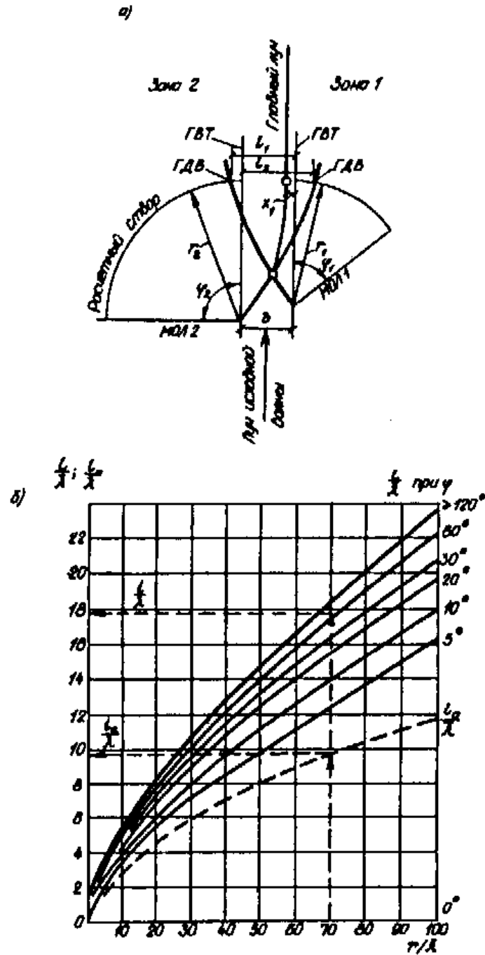
Рис. 9. Схема (а) и графики (б) для определения величин i и l_\alpha
