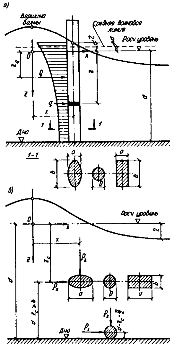
Рис. 14. Схемы к определению волновых нагрузок на обтекаемые преграды а - вертикальные; б - горизонтальные
