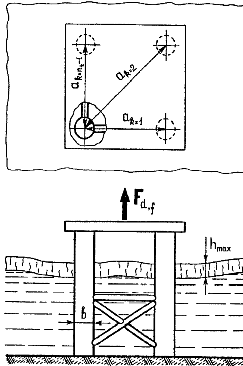
Рис. 43. Схемы приложения нагрузки от примерзшего к сооружению из системы вертикальных колонн ледяного покрова при повышении уровня воды
