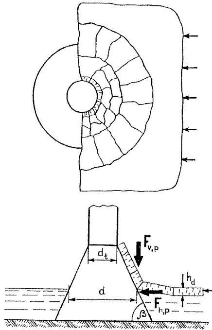
Рис. 37. Схема приложения нагрузок от движущегося ледяного поля на отдельно стоящую коническую опору
