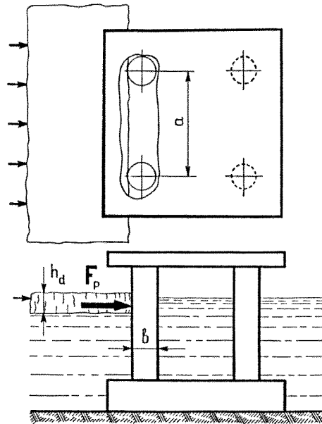
Рис. 39. Схема приложения нагрузок от движущегося ледяного поля на сооружение из системы вертикальных колонн
