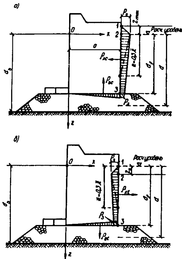
Рис. 6. Эпюры давления дифрагированных волн на вертикальную стену со стороны огражденной акватории
