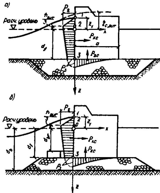
Рис. 9. Эпюры давления прибойных волн на вертикальную стену а - с верхом постели на уровне дна; б - с возвышающейся над дном постелью
