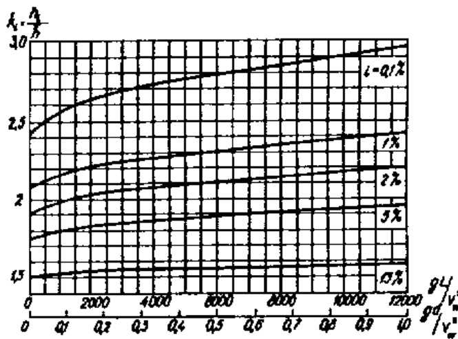
Рис. 2. Графики значений коэффициента k_i
