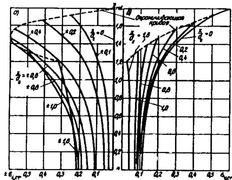
Рис. 25. Графики значений инерционного \varepsilon_{i,cr} и скоростного \varepsilon_{v,cr} коэффициентов НАГРУЗКИ ОТ ВОЛН НА СКВОЗНОЕ СООРУЖЕНИЕ ИЗ ОБТЕКАЕМЫХ ЭЛЕМЕНТОВ
