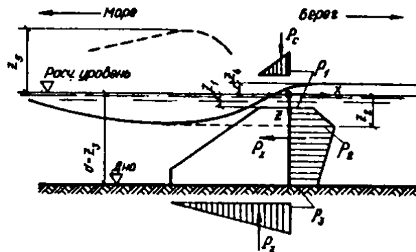
Рис. 26. Эпюры волнового давления на подводный волнолом
