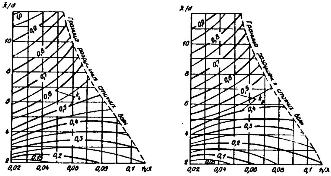
Рис. 4. Графики значений коэффициентов k_4 и k_5
