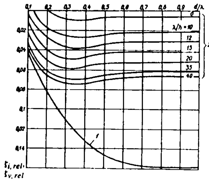
Рис. 21. Графики значений относительных координат
