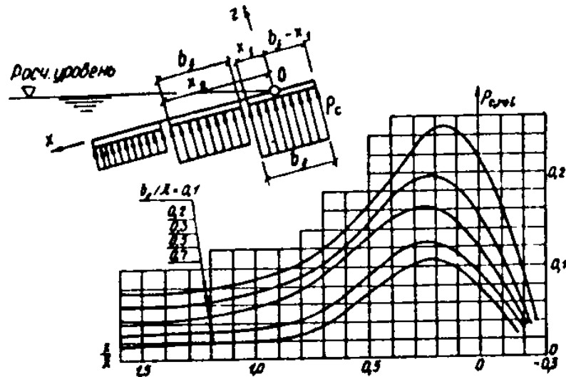
Рис. 12. Графики для определения относительного волнового противодействия
