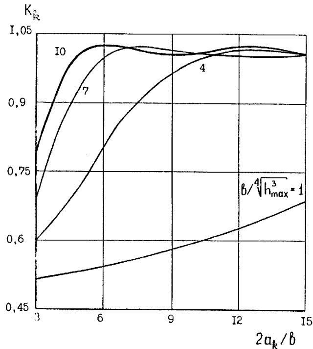
Рис. 44. Графики значений коэффициента K_k
