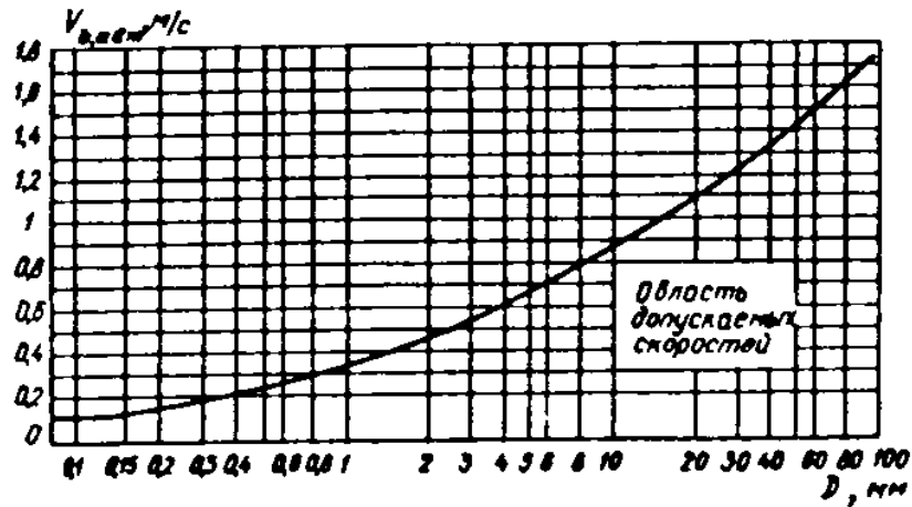
Рис. 7. График допустимых значений неразмывающих донных скоростей
