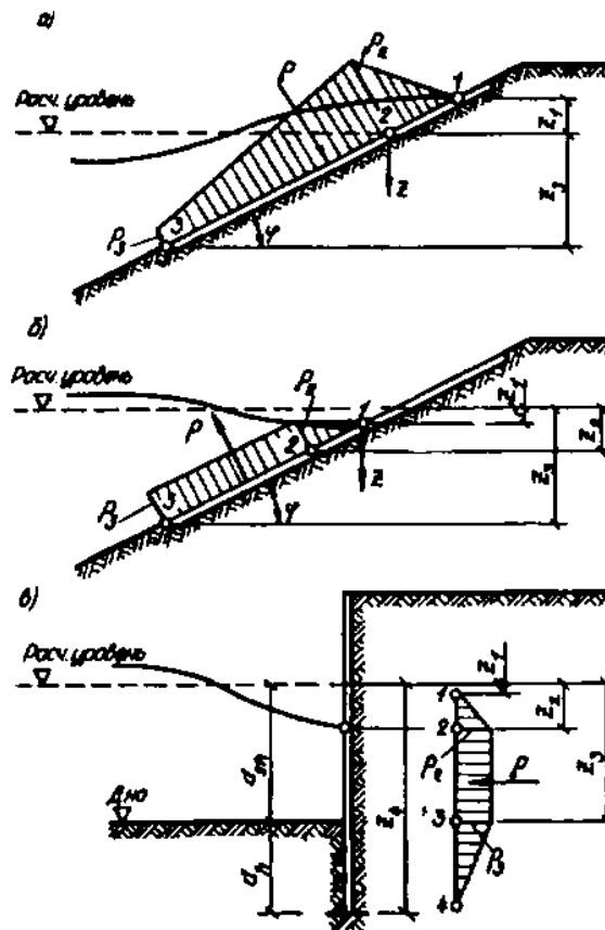
Рис. 31. Эпюры давления судовых волн на укрепления берегов каналов
