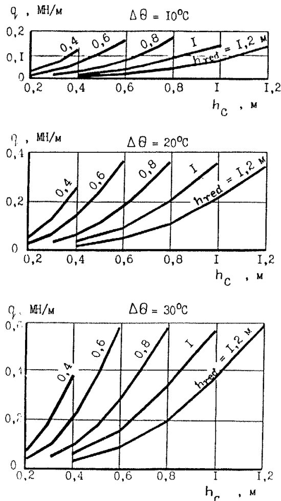
Рис. 40. График значений нагрузки q
