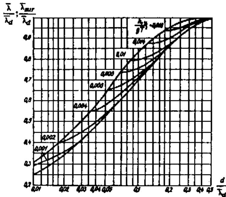
Рис. 4. Графики для определения значений \frac{\bar{\lambda}}{\lambda_d} в мелководной и \frac{\bar{\lambda}_{sur}}{\bar{\lambda}_d} в прибойной зонах
