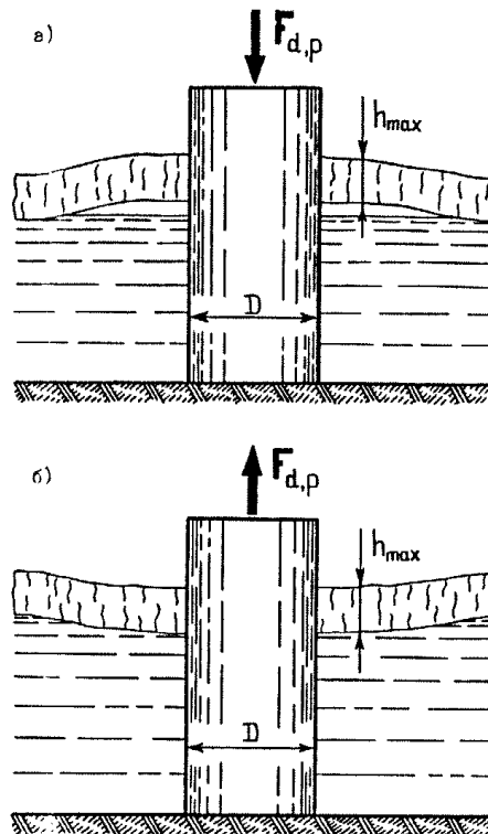
Рис. 41. Схема приложения нагрузок от примерзшего к сооружению ледяного покрова при изменении уровня воды (УВ)
