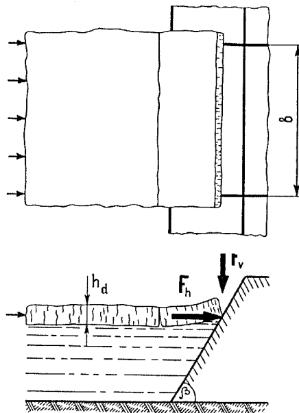
Рис. 38. Схема приложения нагрузок от движущегося ледяного поля на сооружение откосного профиля
