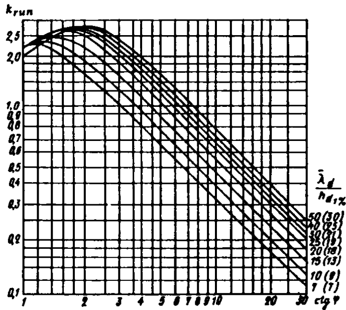
Рис. 10*. Графики значений коэффициента k_{rup}
