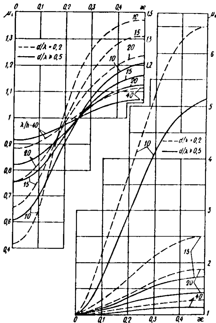
Рис. 22. Графики значений инерционного \mu_i , и скоростного \mu_v коэффициентов фазы НАГРУЗКИ ОТ ВОЛН НА ГОРИЗОНТАЛЬНУЮ ОБТЕКАЕМУЮ ПРЕГРАДУ
