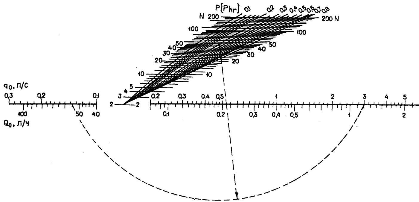
Черт. 3. Номограмма для определения секундных и часовых расходов воды q при q_0 \leq 0,3 л/с, N \leq 200
