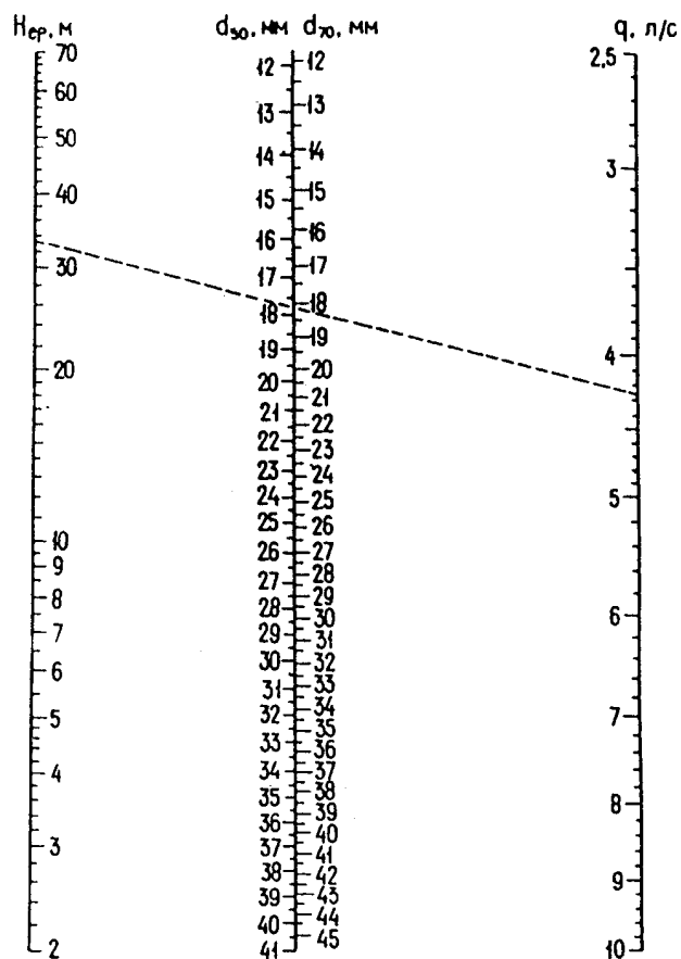
Черт. 5. Номограмма для определения диаметров отверстий диафрагм, устанавливаемых между соединительными головками и пожарными кранами
