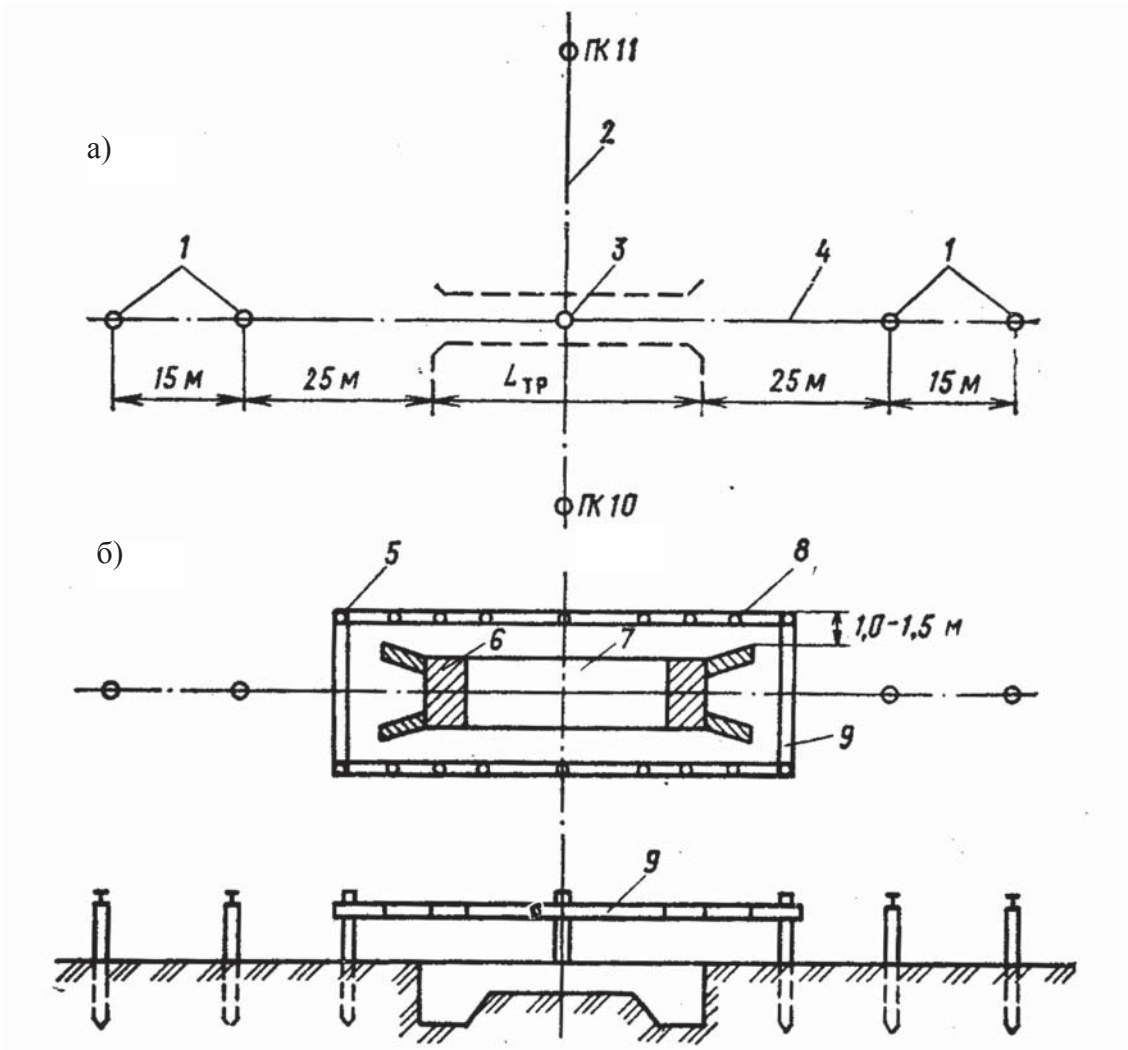
а) разбивка и закрепление осей трубы; б) разбивка котлована 1 – выносные метки (столбы); 2 – ось трассы; 3 – точка пересечения осей трубы и насыпи; 4 – ось трубы; 5 – столб; 6 – оголовок; 7 – котлован; 8 – колья; 9 – обноска из досок; L_{\text{ТР}} – длина труб Рисунок Е.1– Схема геодезической разбивки водопропускной трубы
