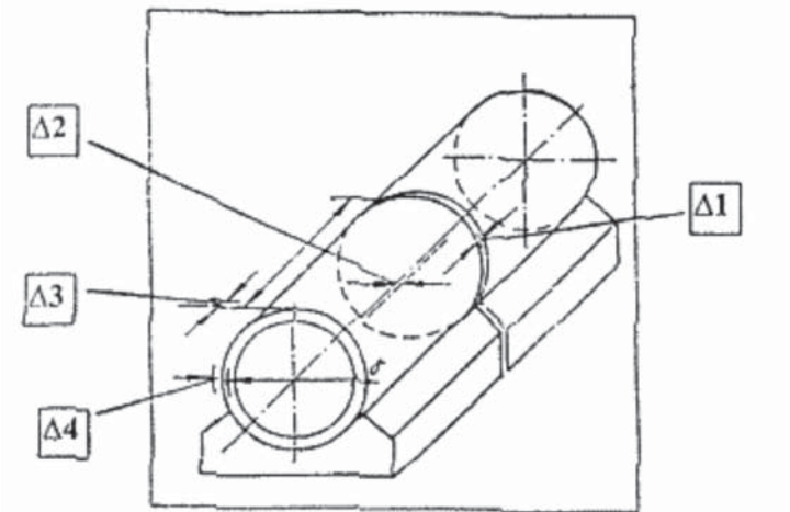
Рисунок К.2 – Круглая железобетонная труба на фундаменте из лекальных блоков
